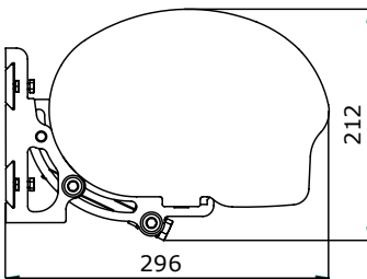
Homlokzati rögzítés
