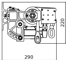
Homlokzati rögzítés
