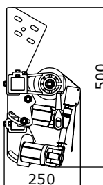
Szarufa rögzítés
