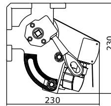
Univerzális rögzítés
