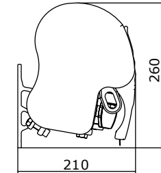
Homlokzati rögzítés
