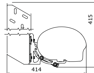
Szarufa rögzítés
